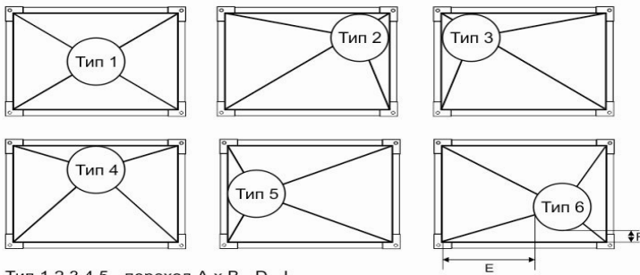
Тип 1,2,3,4,5 - переход А x B - D - L. Тип 6 - переход А x B - D - L (E x F)
