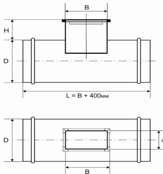
Тройник D x L / A x B - H
