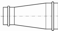
Тип 1 Переход равносторонний. D_1 \times D_2 - L
