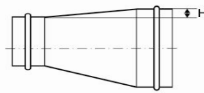
Тип 3 Переход со смещением. D_1 \times D_2 - L (H)
