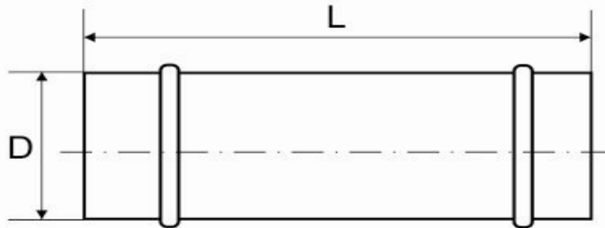
Воздуховод \varnothing D - L
